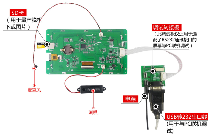
图 1-5 调试工具图
