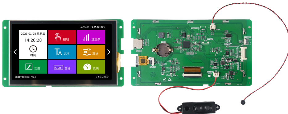
图 1-2 7.0 寸电容触摸参考图
