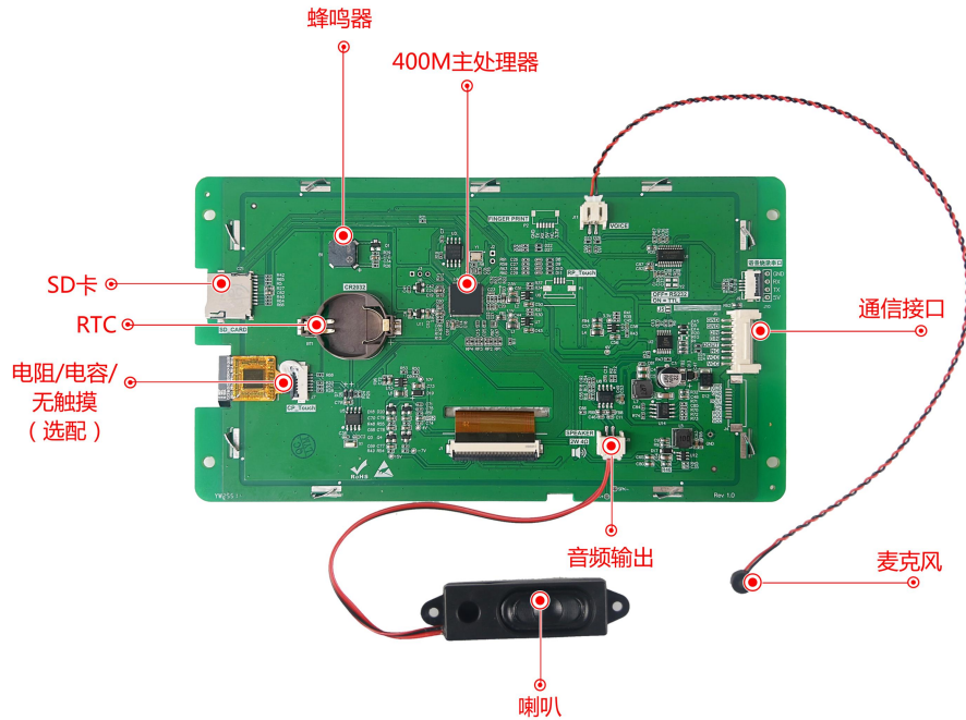
图 1-4 硬件配置图
