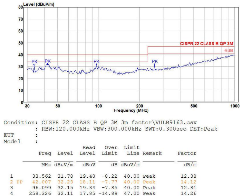
图 4-6 RE 测试垂直方向
